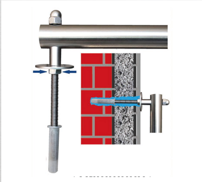
MIT DÄMMUNG
