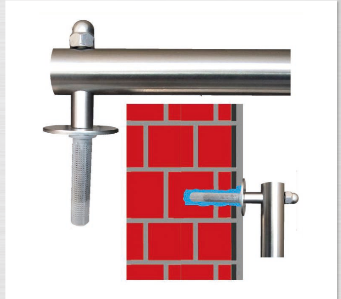
OHNE DÄMMUNG
